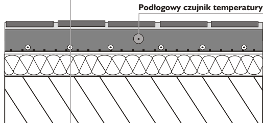
RyS. 3c Przekrój podłogi przy zastosowaniu siatki montażowej
